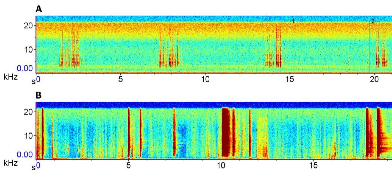
Figura 1. Espectrogramas dos sons A. voluntários e B. estresse produzidos por P. argus
