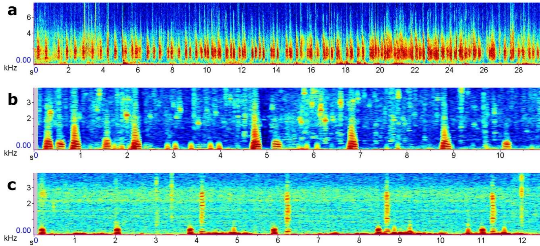
Figura 1. Espectrogramas dos sons de estresse gravados de a. Potamorhina latior e b. Pimelodus blochii , dentro da água quando capturados utilizando rede de emalhe; c. Zungaro Zungaro , fora da água e capturado com espinhel de superfície.
