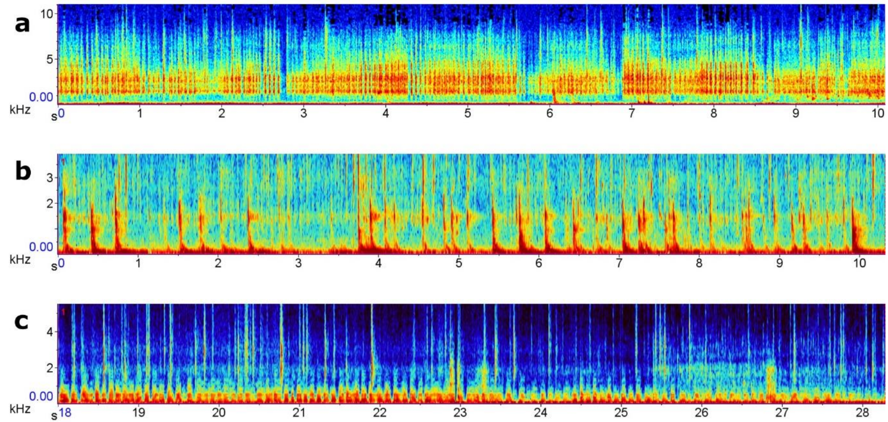
Figura 1. Espectrogramas dos sons detectados no estuário de Maracaípe. a. agregação de caranguejos e b. e c. peixes.
